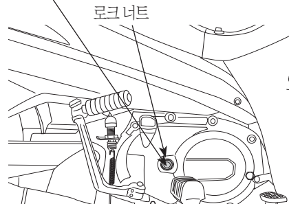
클러치 어저스터
